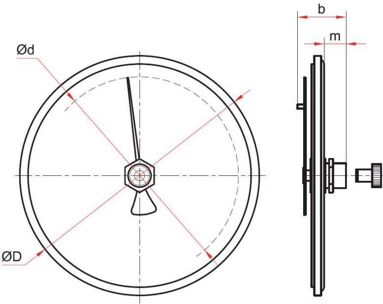
Основные размеры (мм), вес (кг)
